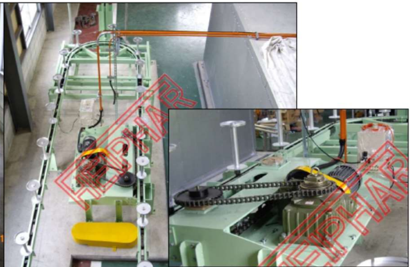
フローコンベアのテークアップ部及び駆動部 テークアップ奥側は前処理装置の下層部アルミ切削粉収集装置及び化成置換槽
